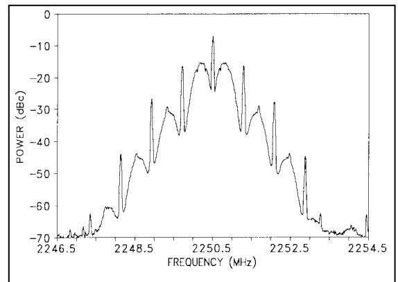
Figure A-4. Bi \phi PCM/PM signal.
